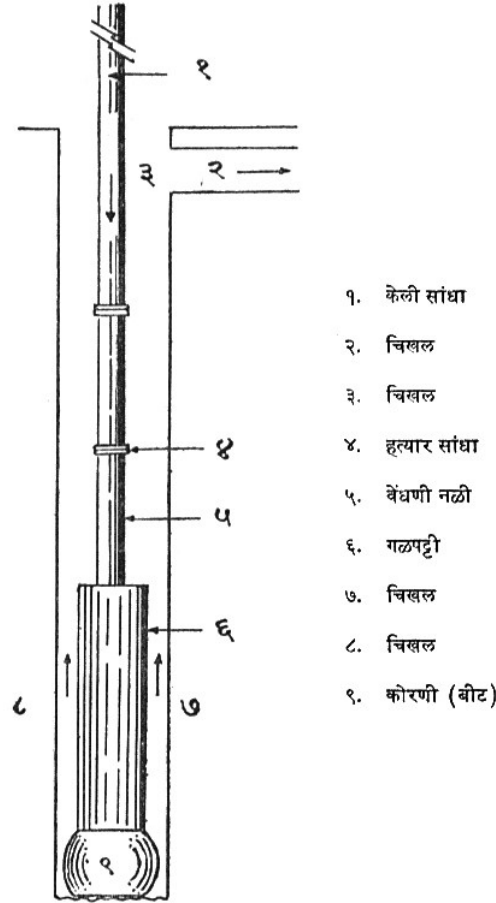
वेधण्याची पद्धत
