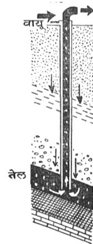
गॅसने तेल काढणे
