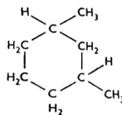
डायमिथिल सायक्लोहेक्सेन
