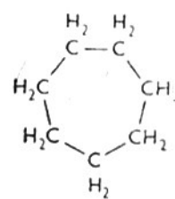
cycloheptane सायक्लोहेप्टेन
