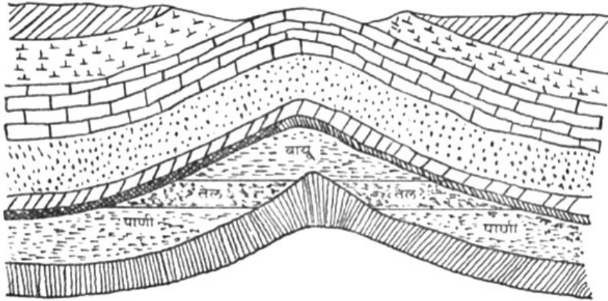
(१) विमुखनति ( anticline)
