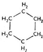
cyclohexane सायक्लोहेक्सेन
