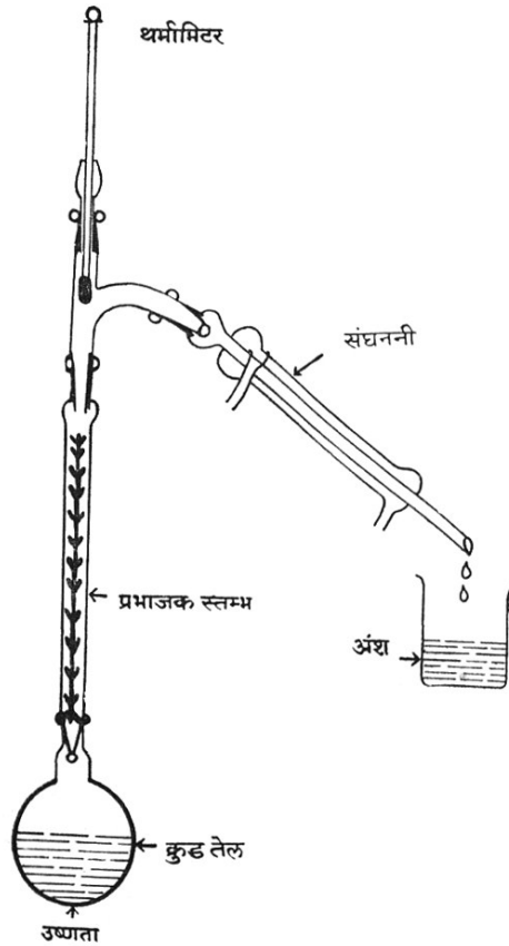
चित्र क्र. ६.२
