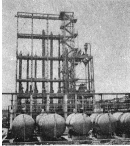
क्लोरोमिथेनचा कारखाना (स्टॅंडर्ड आल्कली, मुंबई)
