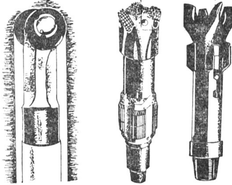
कोरणीचे प्रकार (bits)
