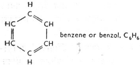
C_6H_6 बेन्झिन
