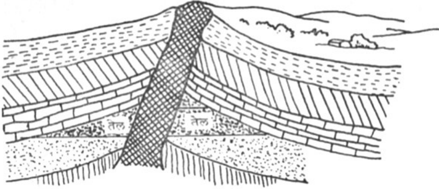
(३) अन्तर्वेशन (intrusion)
