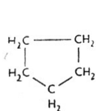
cyclopentane सायक्लोपेंटेन
